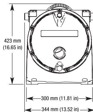
Bombas peristálticas EP3
