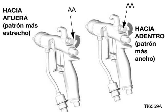
FIG. 5. Perilla de aire del patrón
