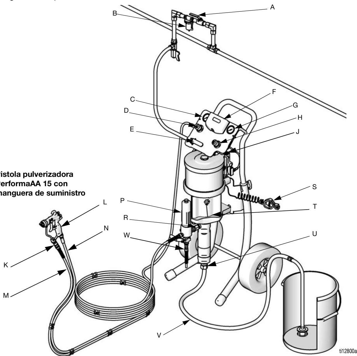
FIG. 1. Instalación típica (su sistema podría no incluir todos los elementos mostrados).
