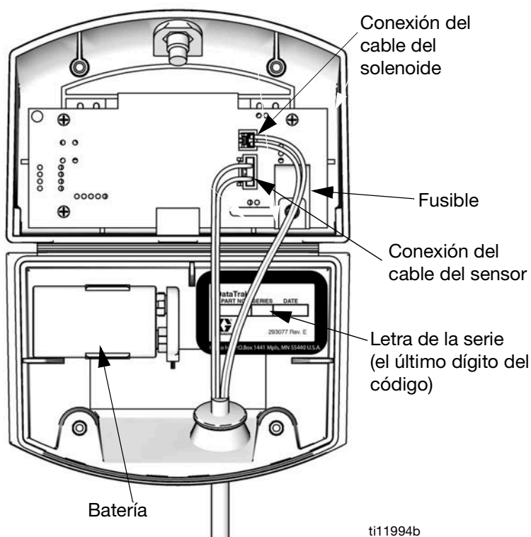
FIG. 11. Ubicación de la pila y el fusible del DataTrak
