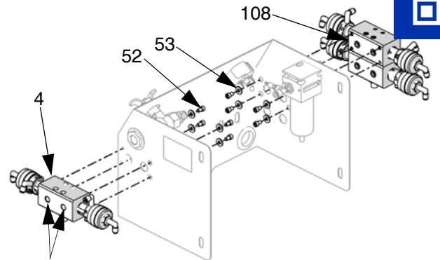
Fig. 22. Desmontaje de las pilas de válvulas
