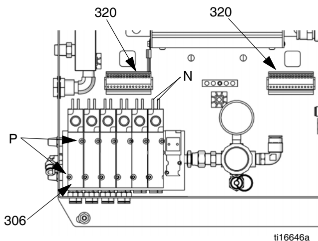
FIG. 3. Reemplazo de una sola electroválvula
