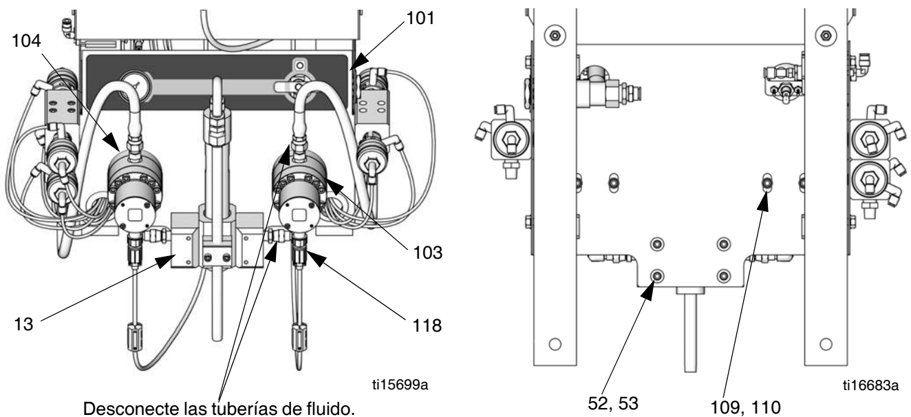
FIG. 24. Desmontaje del colector de sistema c/medidor
