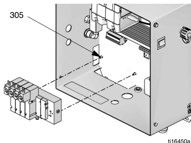
FIG. 4. Reemplazo del módulo de electroválvulas
